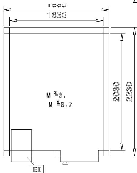
Boven aanzicht
