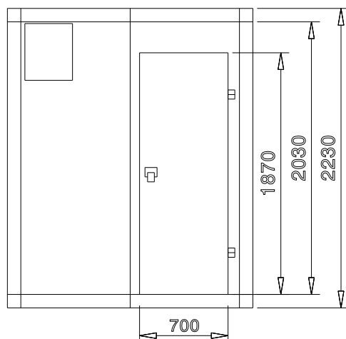
Zij aanzicht
